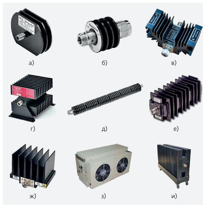
Рис.11. Конструкции коаксиальных фиксированных аттенюаторов большой мощности ( P_{\text{вх.}} > 2 Вт): а – модель 75А, 5 Вт (Weinschel); б – модель 23, 10 Вт (Weinschel); в – RFS50GXD, 50 Вт (RF-Lambda); г – серия 770, 100 Вт (Narda Microwave-East); д – модель 66, 150 Вт (Weinschel); е – модель 58, 250 Вт (Weinschel); ж – серия 300-WA, 300 Вт (Bird Technologies); з – серия RFS800G, 800 Вт (RF-Lambda); и – RFS2000G3, 2000 Вт (RF-Lambda)
