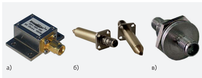
Рис.10. Фланцевые модели коаксиальных аттенюаторов различных производителей: а – 551-199-100 (Broadwave Technologies); б – HFS-835 (Ingun), в – RFS2G18F (RF-Lambda)
