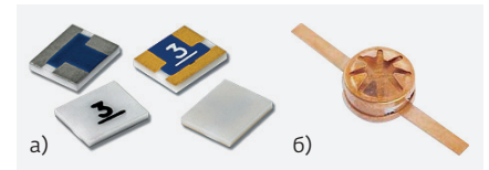
Рис.3. Варианты конструктивного исполнения фиксированных аттенуаторов малой мощности: а – flip-chip (серия TS03, EMC Technology RF Labs); б – pill (серия PSA, Weinschel)
