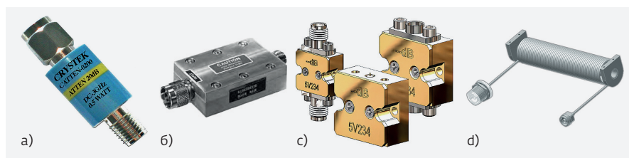
Рис.7. Варианты конструктивного исполнения коаксиальных фиксированных аттенюаторов: а – трубчатый корпус (Crystek); б – прямоугольный корпус (Weinschel); в – drop-in исполнение, дополняемое при необходимости коаксиальными соединителями (AKON); г – на кабельных сборках (R & D Microwave)
